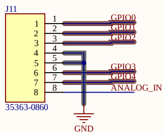
Breakout GPIO (1x8)
