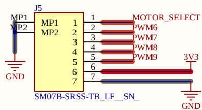
ESC Connector (1x7)
