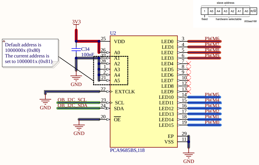
PCA9685
