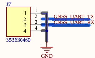
GNSS UART (1x4)
